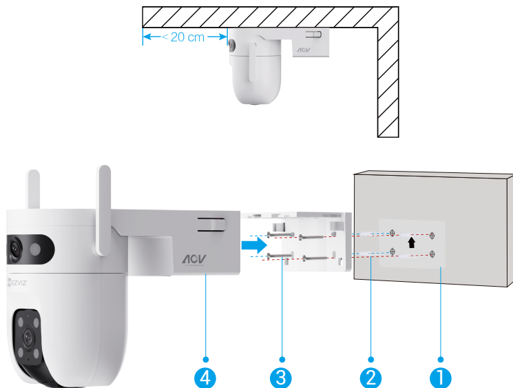
Fig. 2 Vägghermontering
