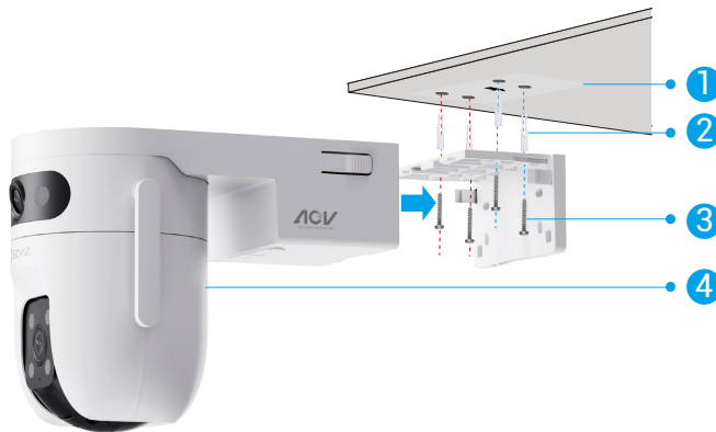
Fig. 1 Takmontering
